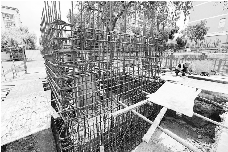
程同时预留东区第二污水通道南延接驳口,远期将石狮八七路DN800污水管接入东区第二污水通道,优化东沟上游污水系统布局。
