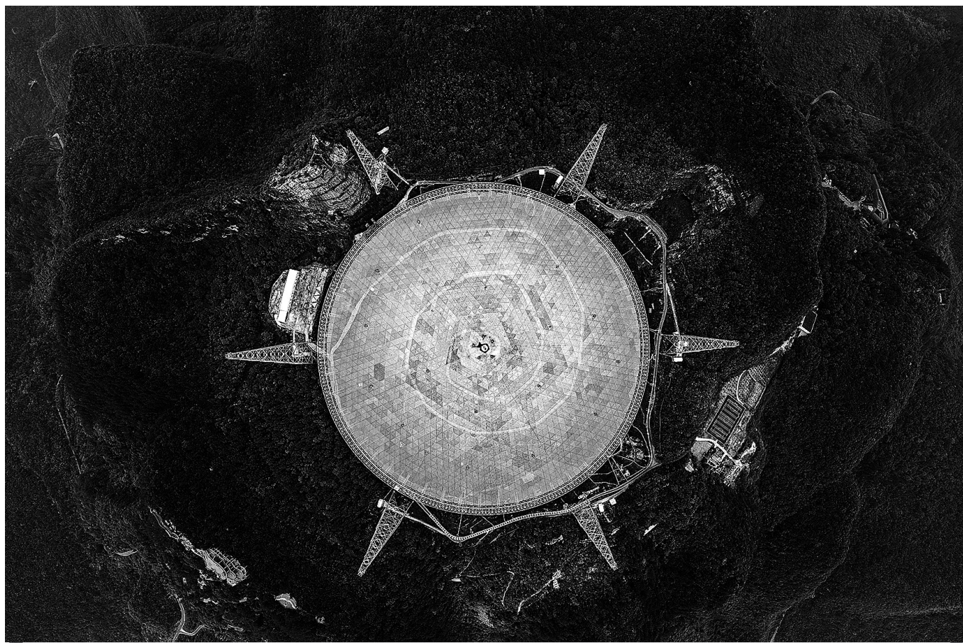
▲“中国天眼”关键部件实现“中国造” 5月6日拍摄的“中国天眼”全景(无人机全景照片,维护保养期间拍摄)。近日,被誉为“中国天眼”的500米口径球面射电望远镜启动馈源驱动钢丝绳更换工作。“中国天眼”的馈源舱重达30吨,6根钢丝绳能以极高精度牵引这只“眼球”,在140米高空、206米尺度范围内实现实时定位,被称为“中国天眼”的“眼部肌肉”。此前该部件依赖进口,2023年1月研发团队启动自主研发,经3轮迭代、6.2万次滑轮运行及20万次脉冲疲劳试验,于2025年8月成功实现国产化。目前6根国产钢丝绳已运抵现场,更换工作预计持续至6月下旬。此次国产化替代不仅解决了供应链安全问题,更建立了从材料、制绳、评价到检测的完整技术体系,为其他重大科技基础设施的国产化提供了可复制的经验。(新华社)
